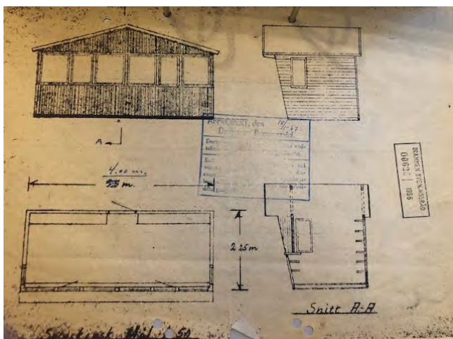
Tegninger av «Rorbua»
