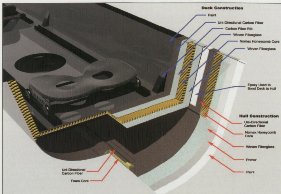
Figuren viser konstruksjon av 1x scullerskrog (Wintech competitor).
