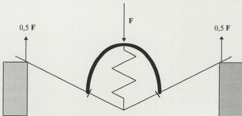
Figur 2 Mekanisk modell av robåt med årer
